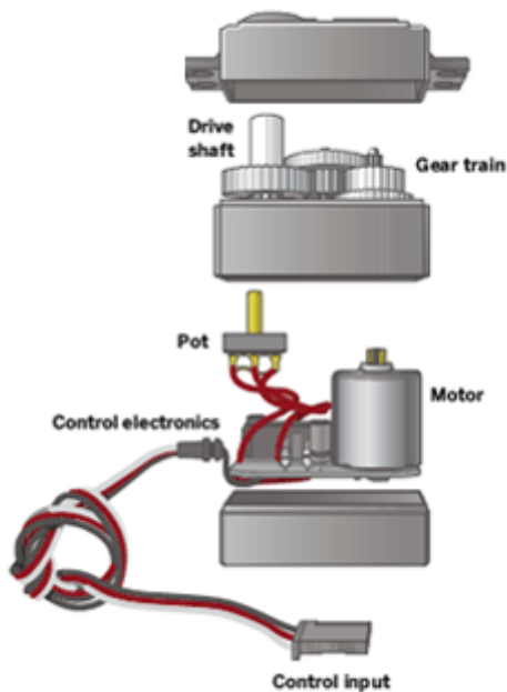
Figura 7. Funcionamento de um servo motor.
