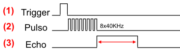
Figura 5. Processo de funcionamento do sensor de ultrassom.
