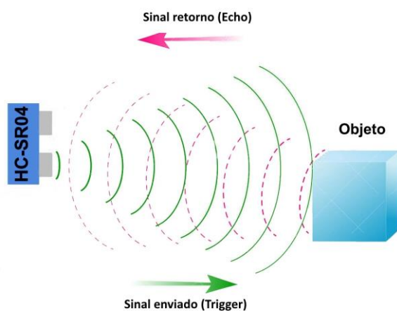
Figura 4. Processo de funcionamento do sensor de ultrassom.
