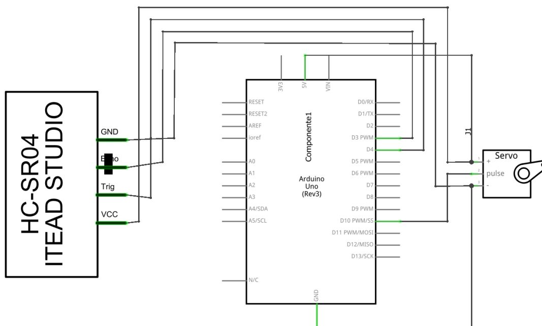
Figura 8. Circuito digital de controle.
