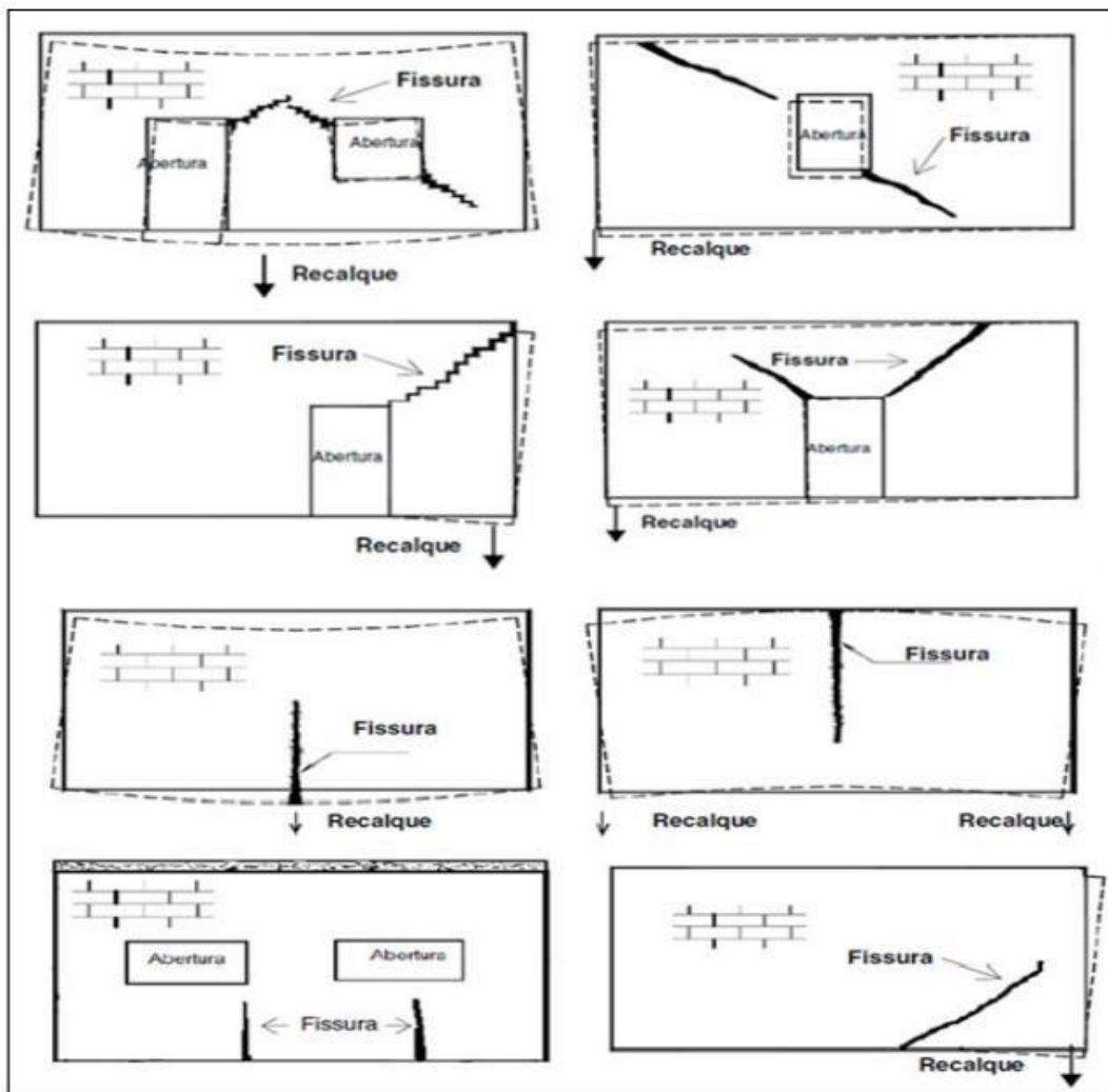
FIGURA 04- Tipos de recalques.
