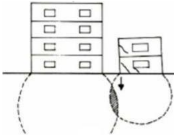
FIGURA 02- Fundações vizinhas gerando um bulbo de tensão a fundação da edificação.
