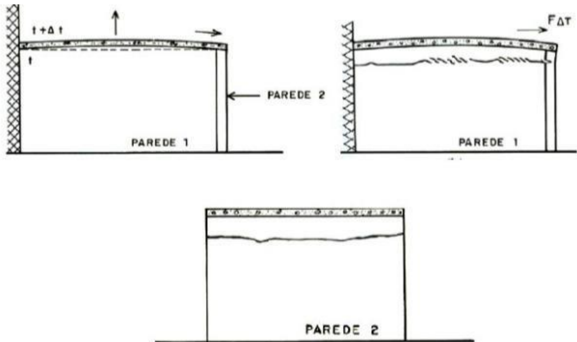
FIGURA 05- Anomalias referente a dilatação térmica.
